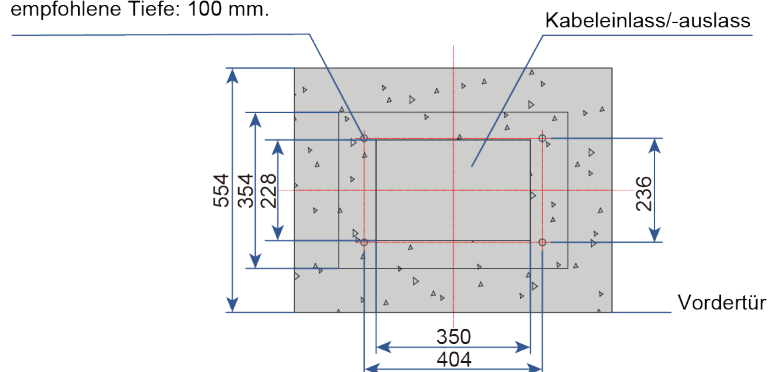
Abbildung 3-4 Lage der Bohrungen für Dehnschrauben
