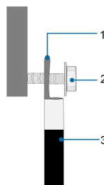
Abbildung 3-5 Aluminiumkabel-Anschluss
