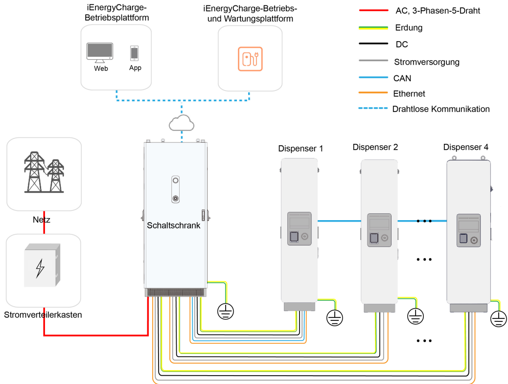
Abbildung 2-1 Systemschaltplan
