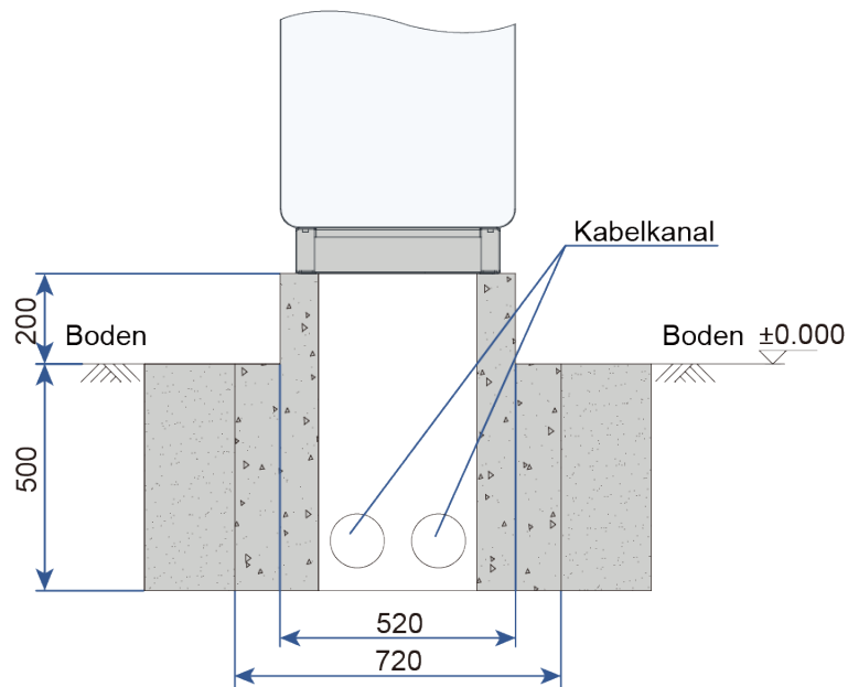
Abbildung 3-3 Abmessungen des Fundaments (mm)
