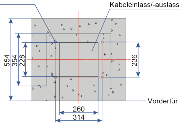
Abbildung 3-4 Lage der Bohrungen für Dehnschrauben
