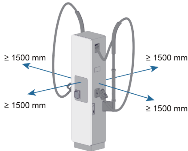
Abbildung 3-1 Platzbedarf für die Installation
