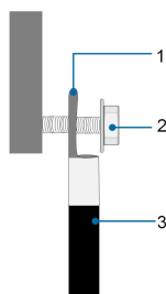
Abbildung 3-5 Aluminiumkabel-Anschluss
