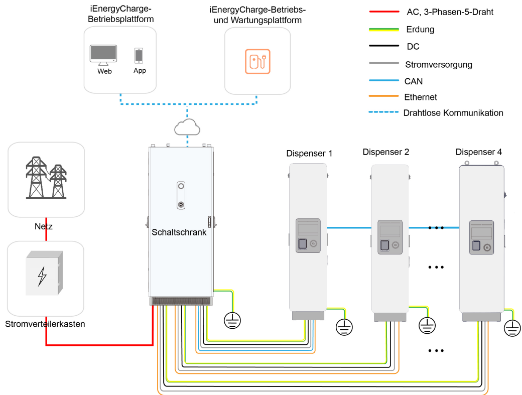
Abbildung 2-1 Systemschaltplan
