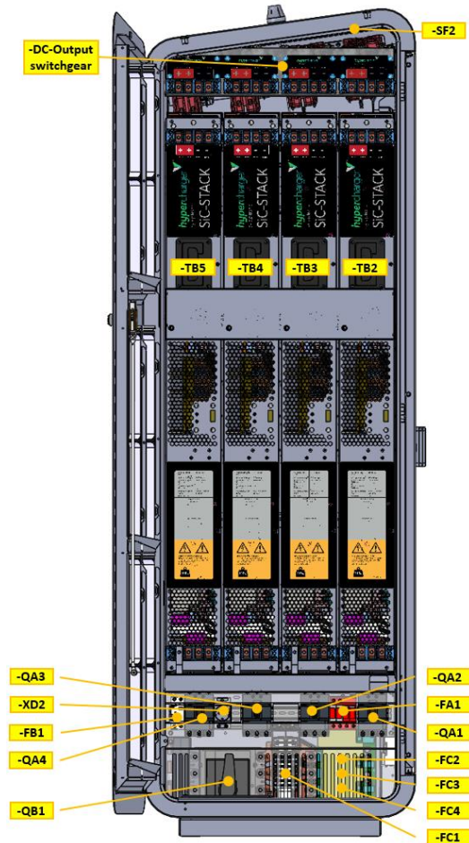
Abbildung 15: Innenansicht (Servicetür-Seite)
