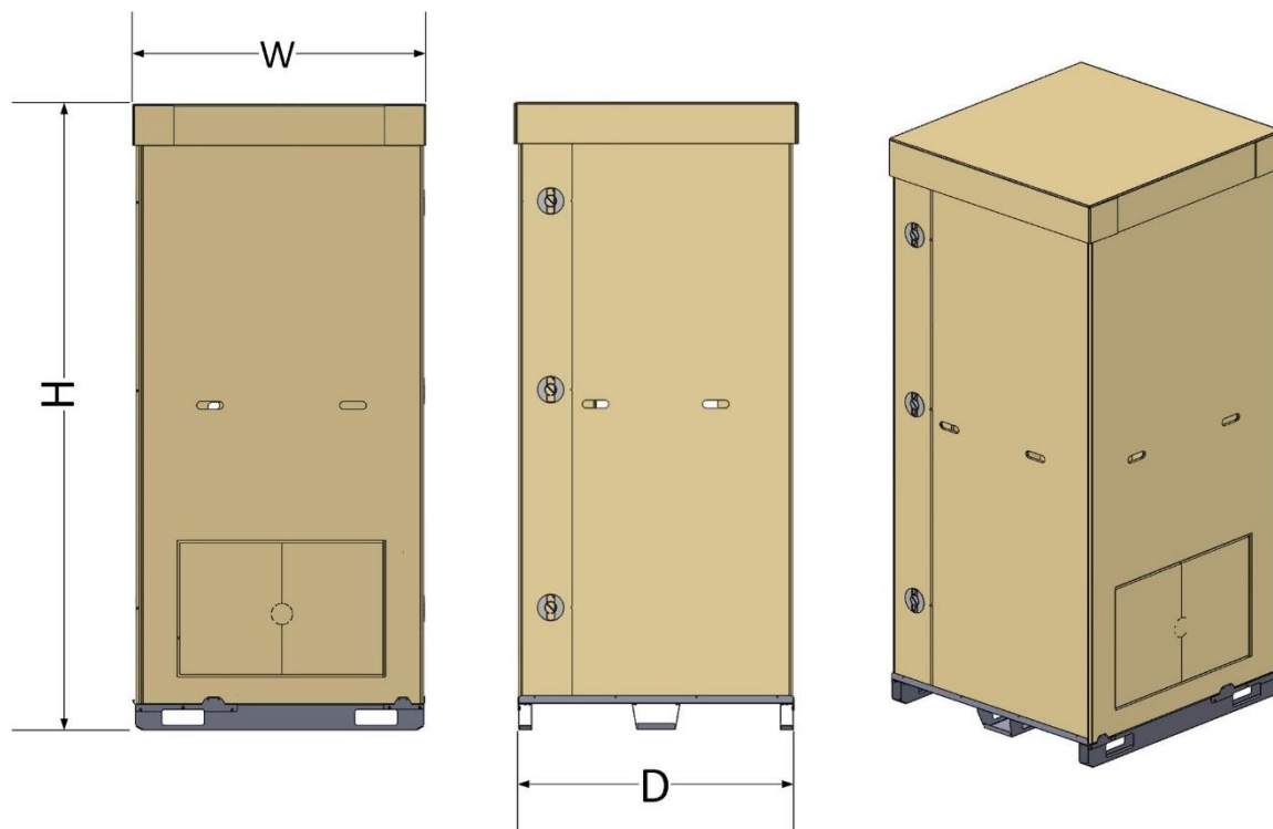
Abbildung 33: HYC400 Kartonverpackung
