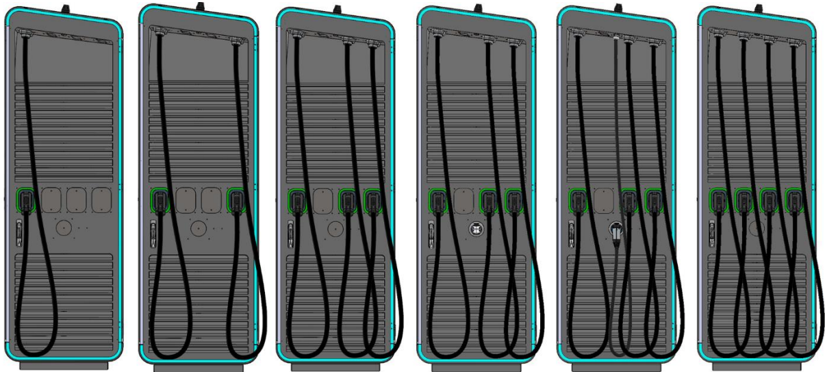
Abbildung 2: Ausstattung Ladeschnittstellen
