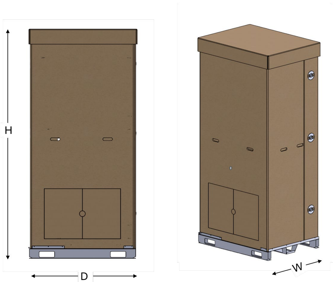
Abbildung 38: HYP200-Kartonverpackung
