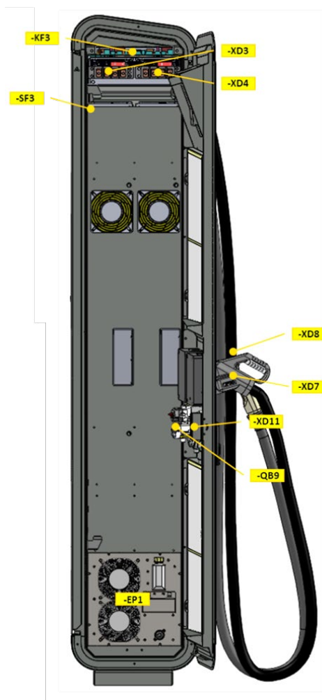
Abbildung 17: Innenansicht (Ladekabeltür-Seite)
