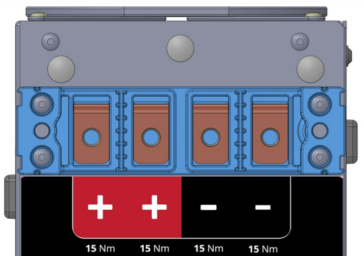
Abbildung 25: DC-Anschlussblock
