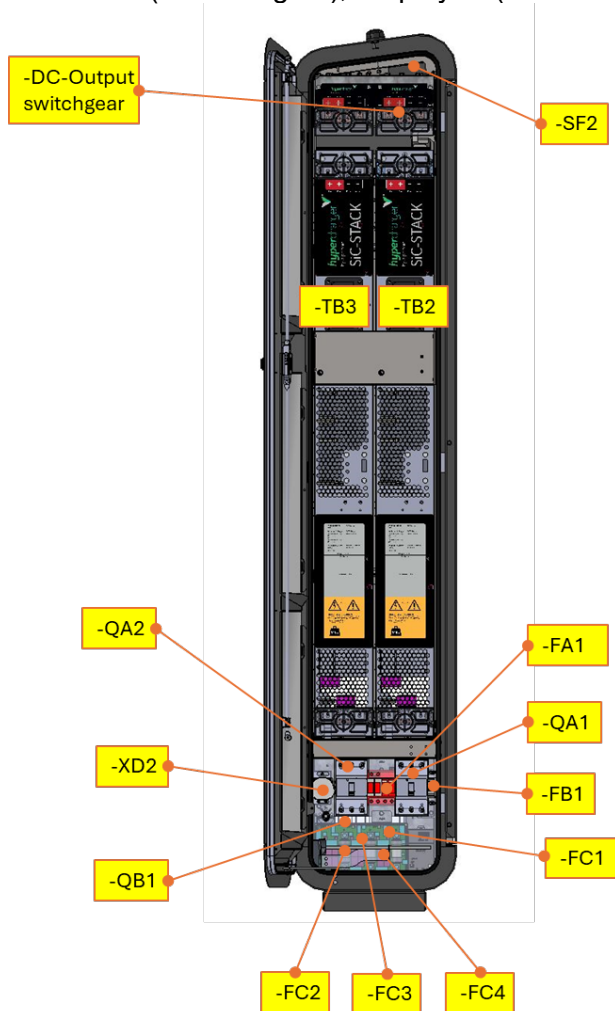
Abbildung 15: Innenansicht (Servicetür-Seite)
