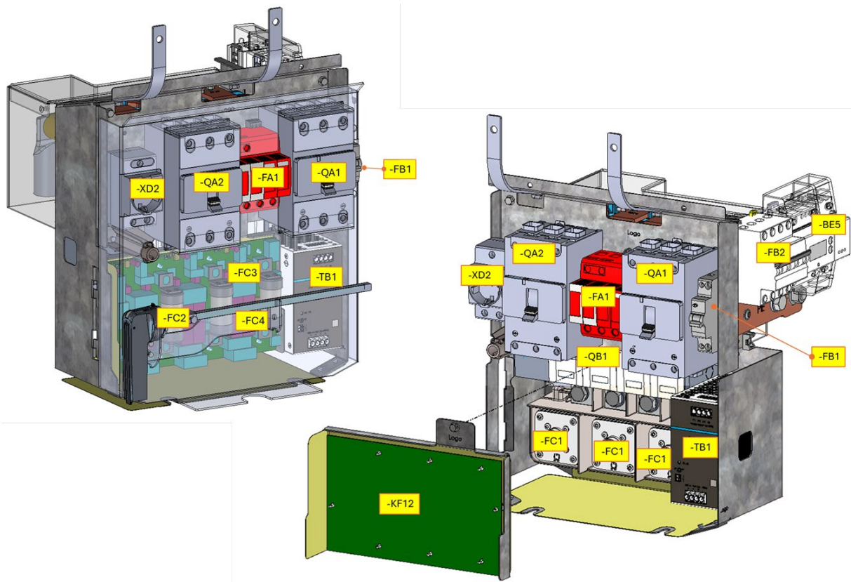
Abbildung 26: AC-Eingangsschaltanlage(Vorderseite)
