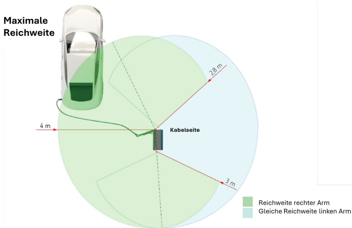
Abbildung 8: Reichweite Kabelmanagement
