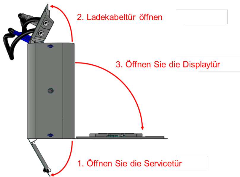
Abbildung 13: Reihenfolge zum Öffnen der Hypercharger-Türen
