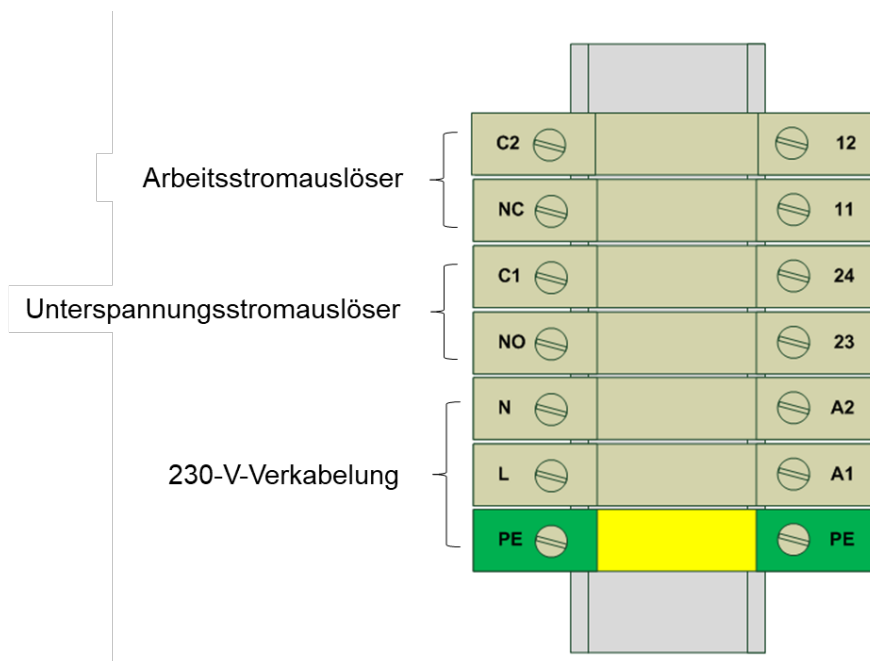
Abbildung 36: Anschlussmöglichkeiten für externes Not-Aus
