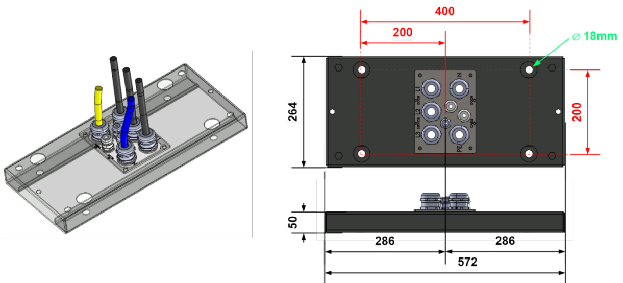
Abbildung 49: HYC200-Sockel inkl. Kabeleinführungsplatte (in mm)
