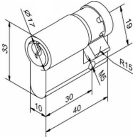
Abbildung 12: Verwendeter Halbzyliner (Angaben in mm)
